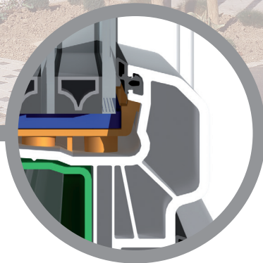
Streamline halb flächenversetzt Streamline semi-recessed
