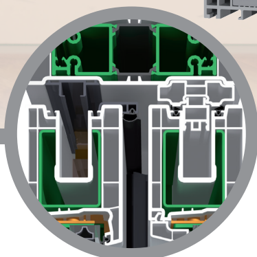
Hebeschiebetür mit Festteil Lift and slide door with fixed panel
